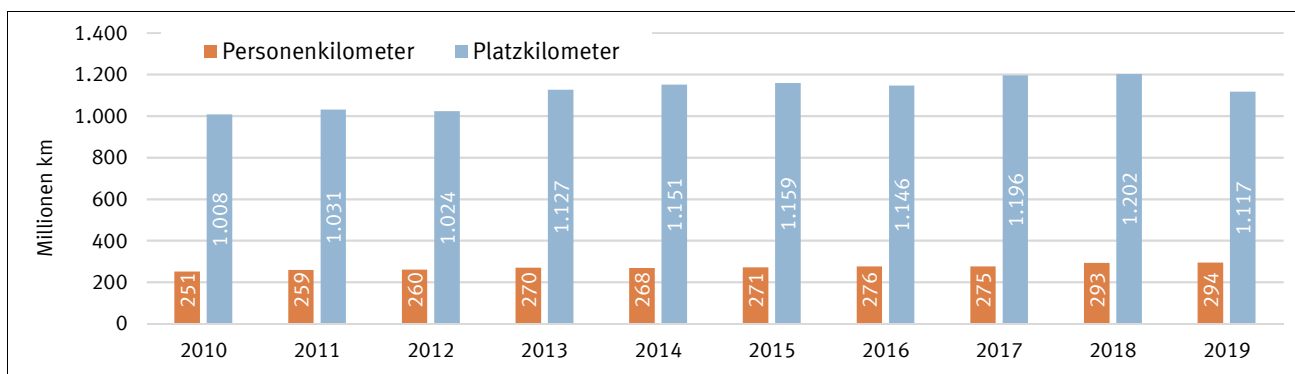
Abb. 5.4 Personen- und Platzkilometer (in Mio.) im Bedienungsbereich der MVG seit 2010
