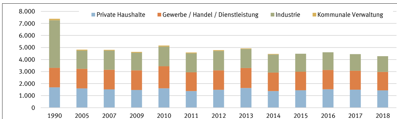
Abb. 6.2 Endenergieverbrauch nach Verbrauchern 1 in Mainz seit 1990 (in GWh/a)
